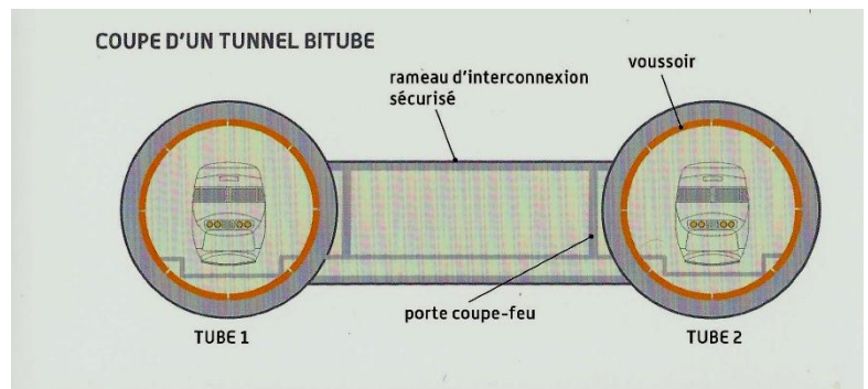
Coupe du tunnel de Saverne (Doc RFF)
