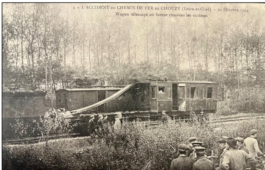
Une des voitures éventrées dans le choc. La structure en bois n'a guère résisté.
